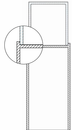
Base rientrata
