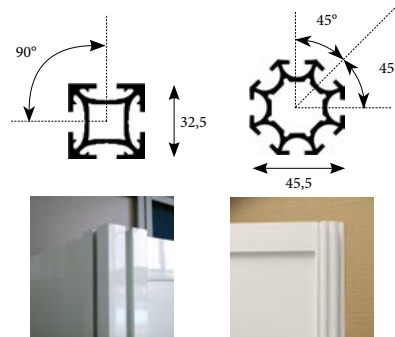
Paletti 4 partenze
