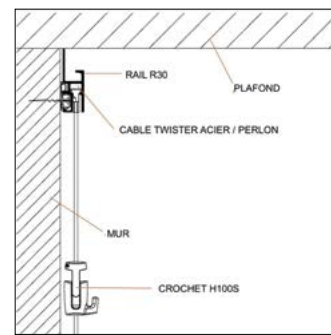
Accrochage par perlon ou câble
